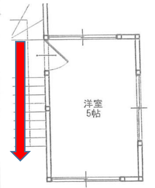
中2階平面図
